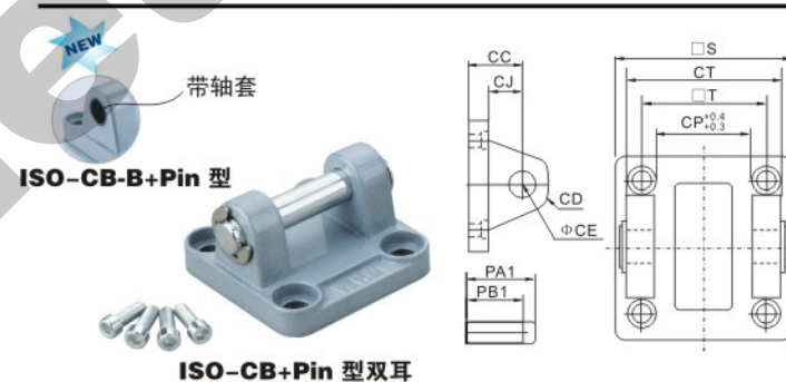
ISO-CB+Pin 型 双耳
