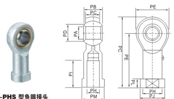
M-PHS 型鱼眼接头
