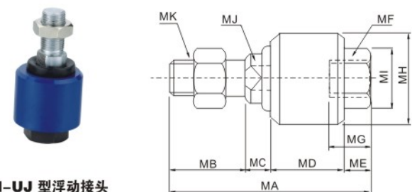
M-UJ 型浮动接头
